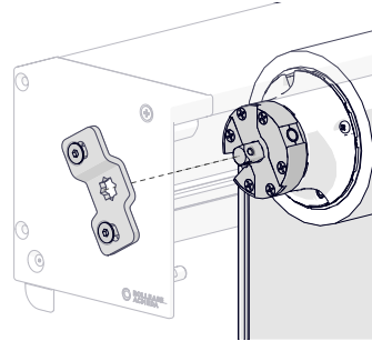
MOTOR
